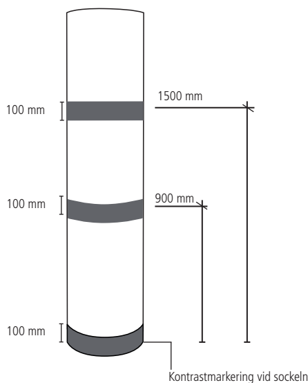
Exempel på kontrastmarkering av pelare eller utstickande byggnadsdelar
