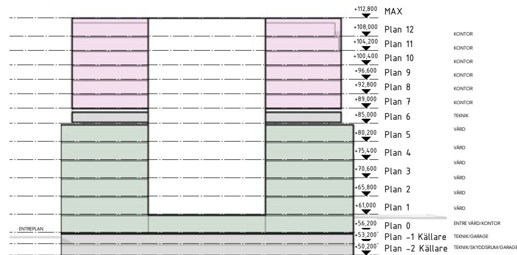
TYPSEKTION 1:1000
