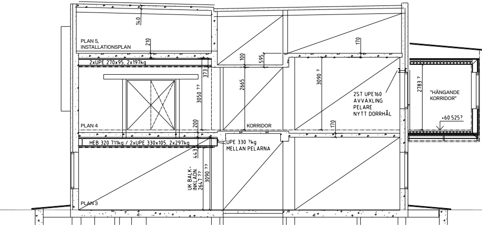
Sektion, påverkan på stommen vid ombyggnad alt. B.
