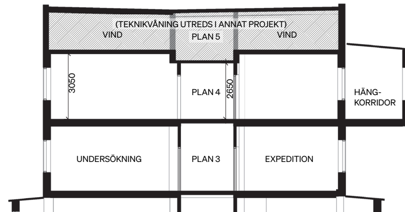
Befintlig sektion A, byggnad 09.
