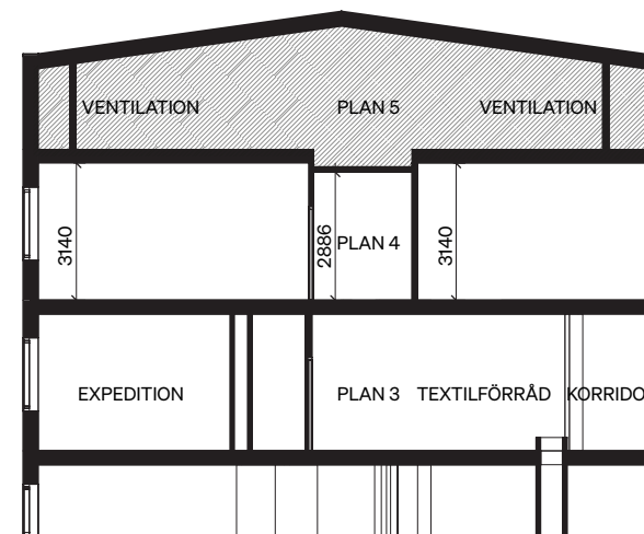
Befintlig sektion D, byggnad 01.
