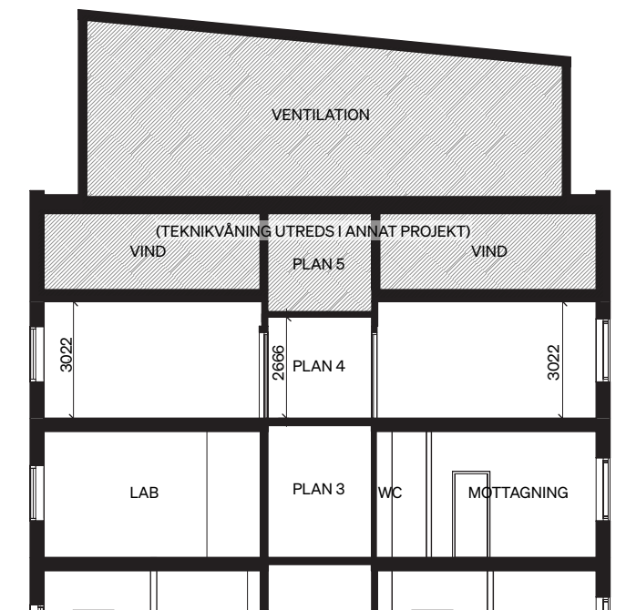
Befintlig sektion C, byggnad 07.
