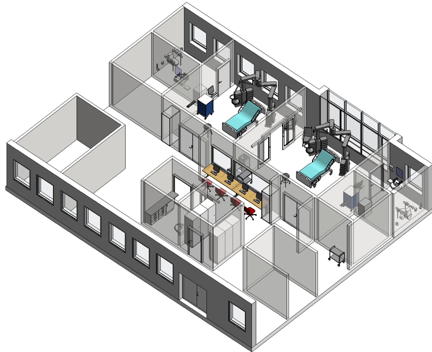
Vårdmodulen i alternativ B, axonometrisk vy
