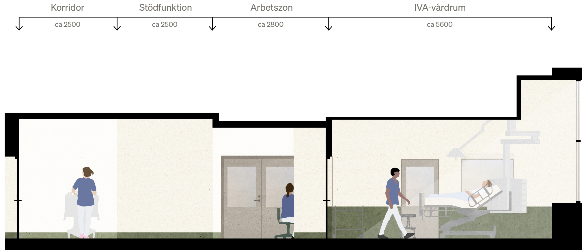
Visionsbild - sektion genom korridor, arbetszon och vårdrum i alternativ B, byggnad 09. Måtten är ungefärliga.
