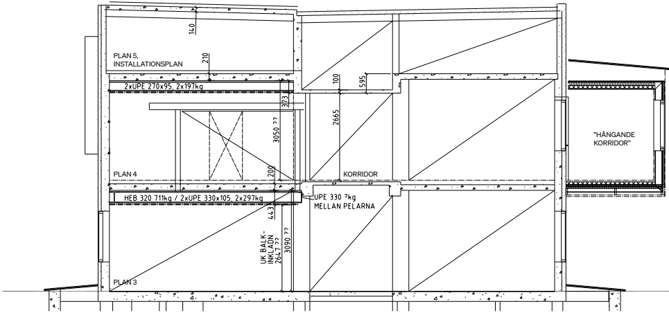
Sektion, påverkan på stommen vid ombyggnad alt. A.
