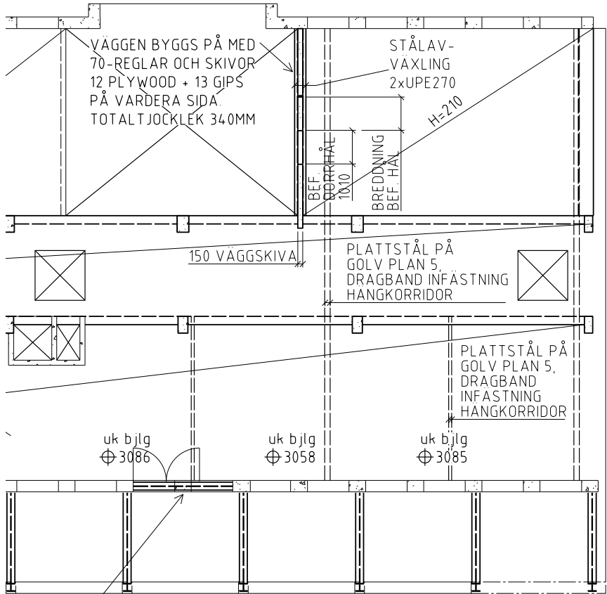
LAYOUT B: DORRLÄGE ANPASSAS, I SIDLED, MOT STOMME KORRIDOR PELARE AVVÄXLAS MED STÅLBALK.
