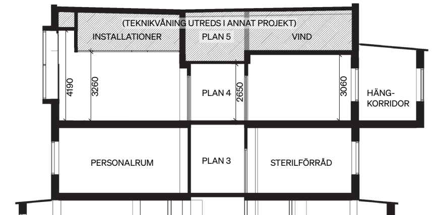
Befintlig sektion B, byggnad 09.
